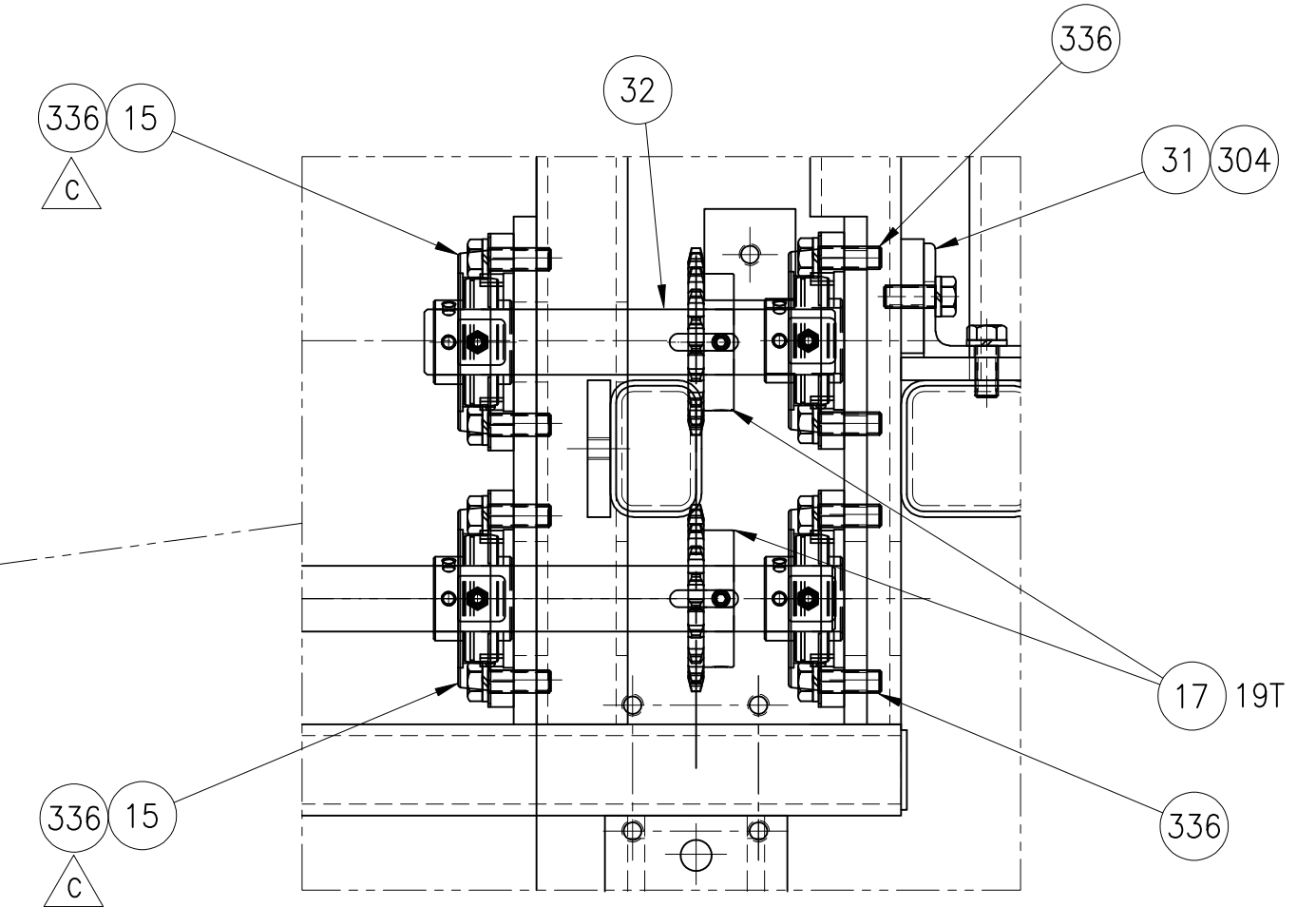
DETAIL VIEW B SCALE: 6" = 1'-0"
